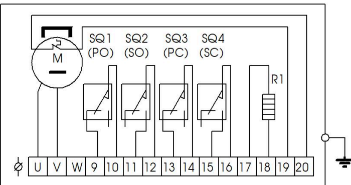
Схема электрическая соединений CE414-1A электропривода непрямоугольного общего промышленного исполнения ГЗ-ОФ (К) типоразмер 8100 питанием DC 24В
