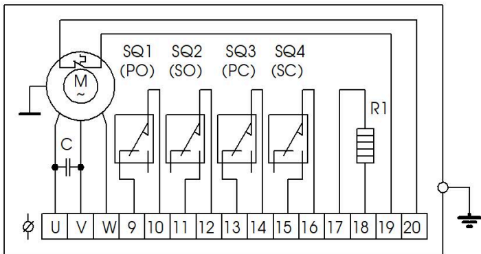
Схема электрическая соединений CE413-7A электропривода непрямоугольного общего промышленного исполнения ГЗ-ОФ (К) типоразмер 8100 питанием AC 230В 50Гц
