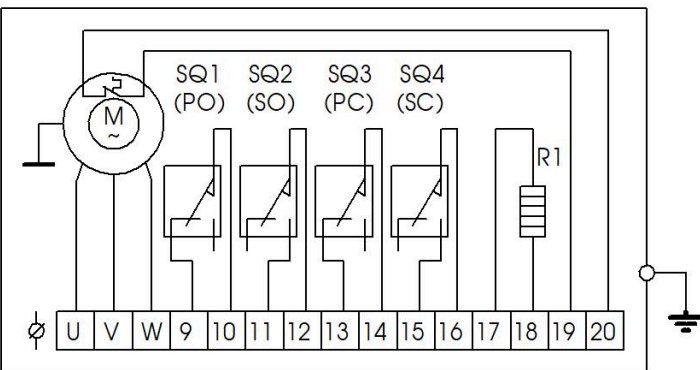
Схема электрическая соединений CE411-7A электропривода непрямоугольного общего промышленного исполнения ГЗ-ОФ (К) типоразмер 8100 питанием 3 AC 400В 50Гц
